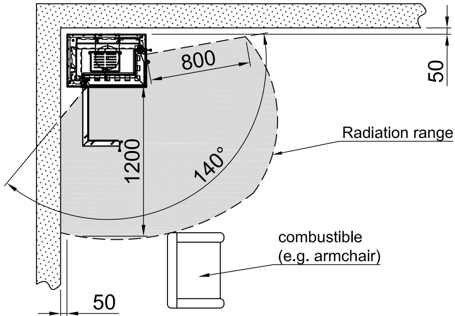
non combustible wall
